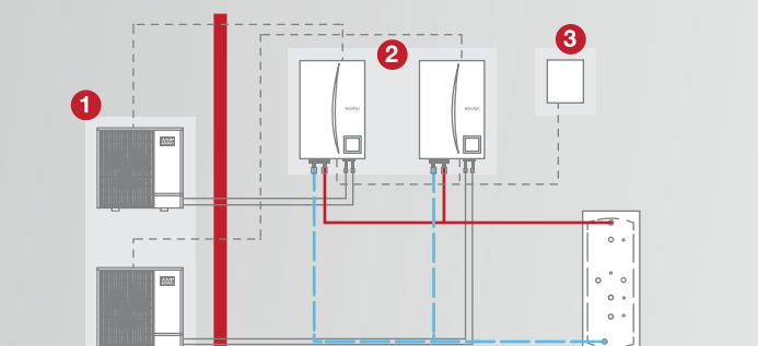
1 Vonkajšie jednotky 2 Hydromodul 3 PAC-IF071
